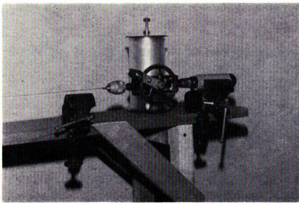
Fig. 3.12. Hand driller.
